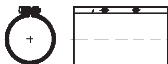
Kabelschale Länge 1m aus Hart-PE rot
